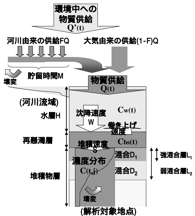
図-2 モデル概要図
