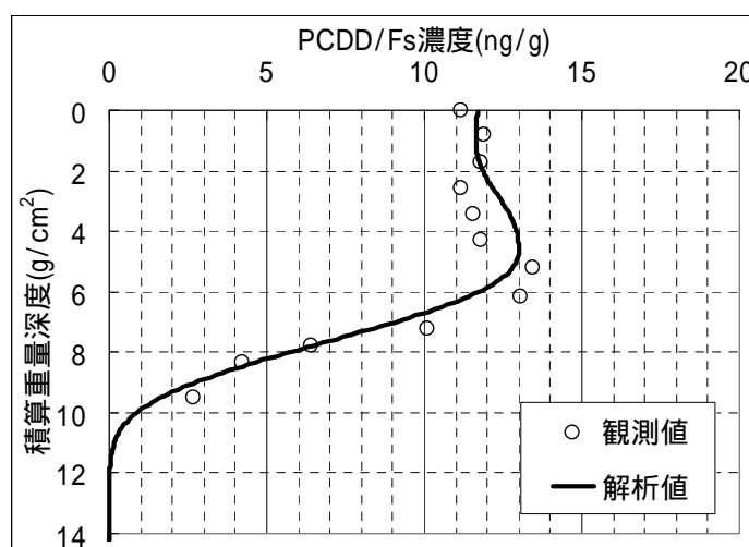
図-5(e) 宍道湖St.40(ダイオキシン類)
