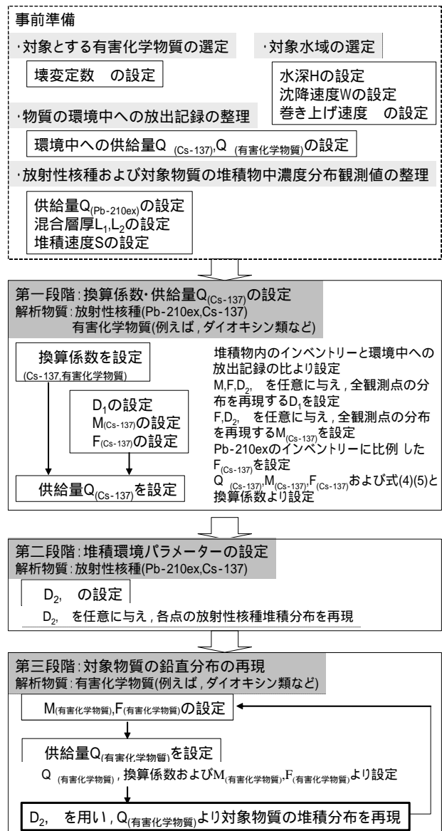
図-3 解析手順
