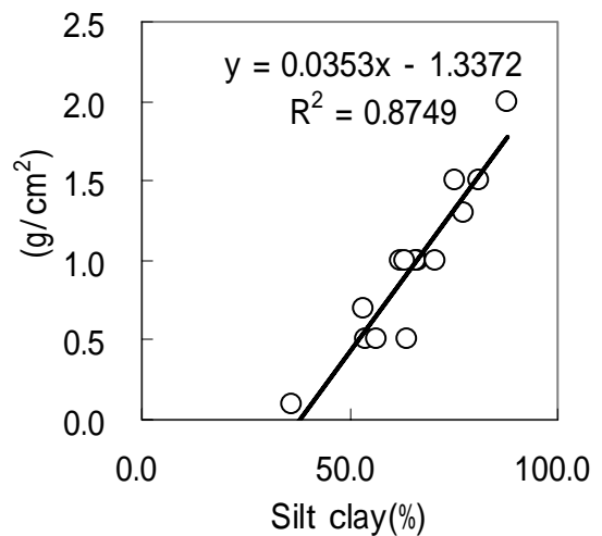
図-6 再懸濁層厚 とシルト粘土含有率の相関
