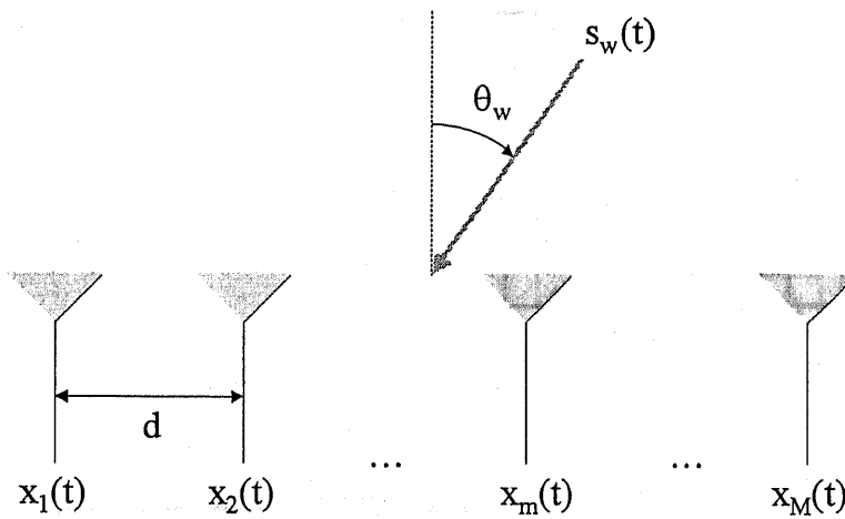
Figure A.3: Array Antenna.
